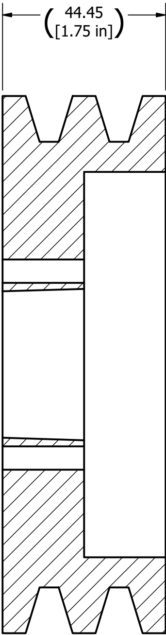
SECTION A-A
