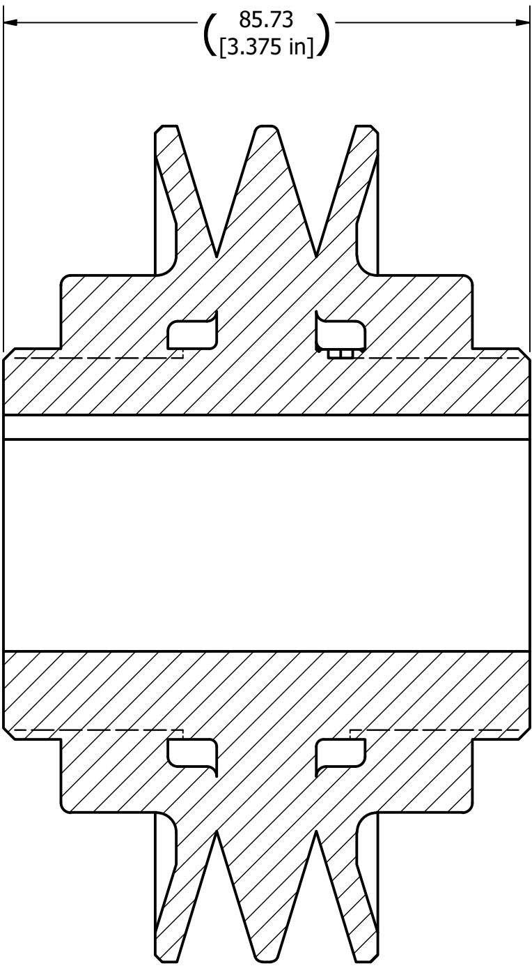
SECTION A-A
