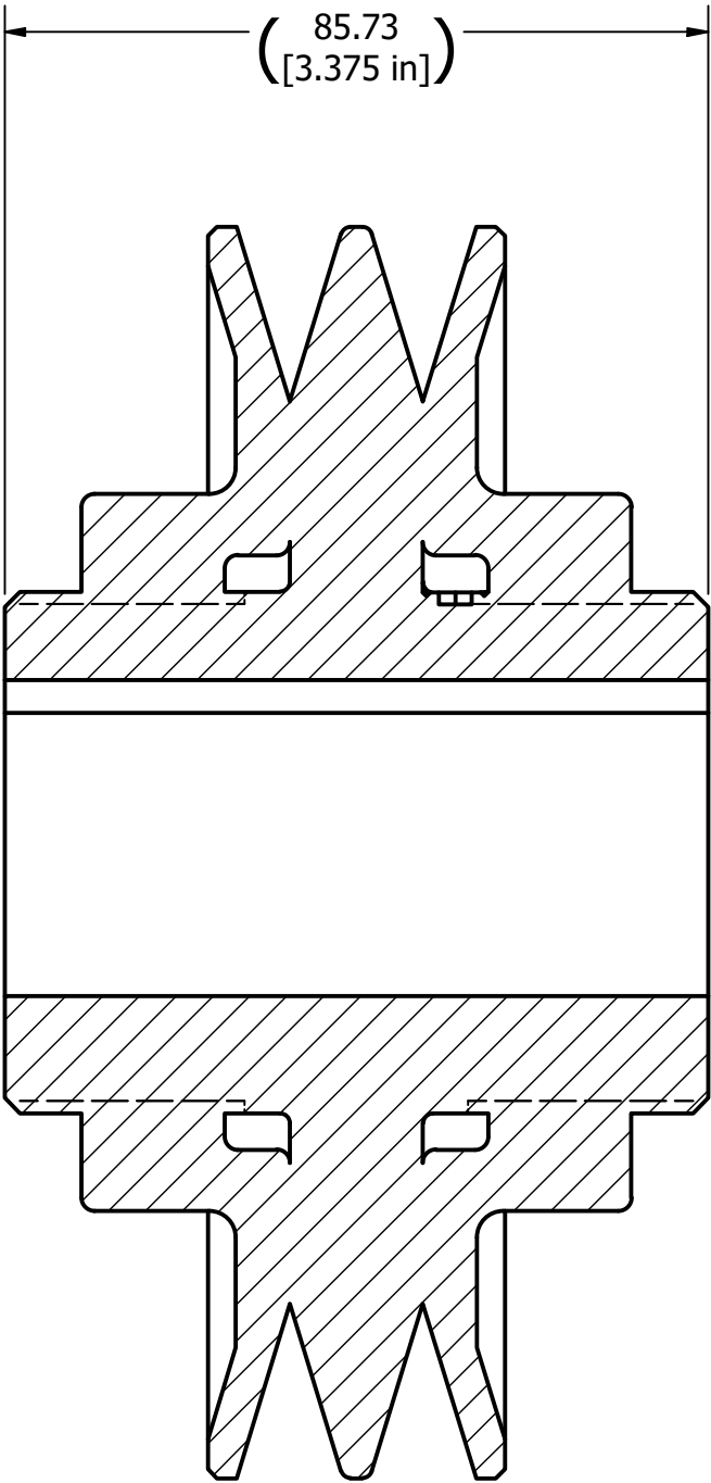
SECTION A-A
