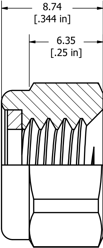
SECTION A-A SCALE 5 : 1
