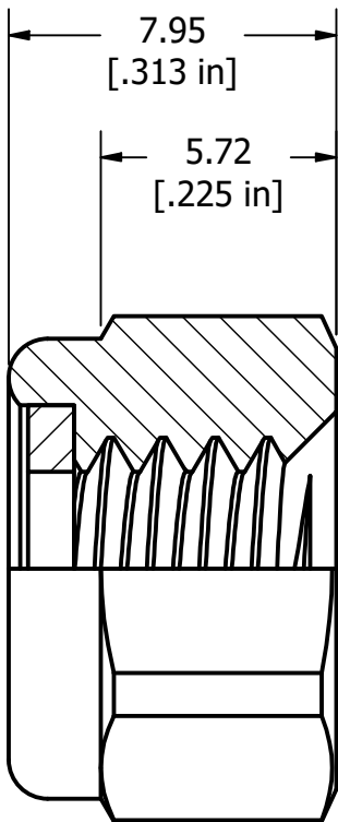
SECTION A-A SCALE 5 : 1
