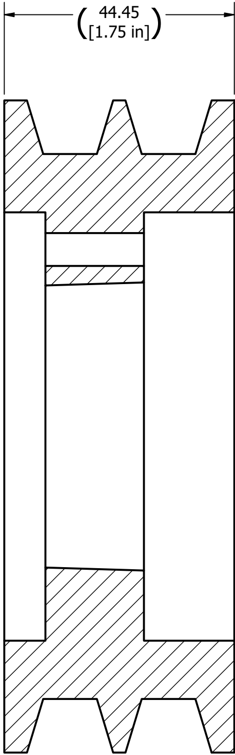
SECTION A-A
