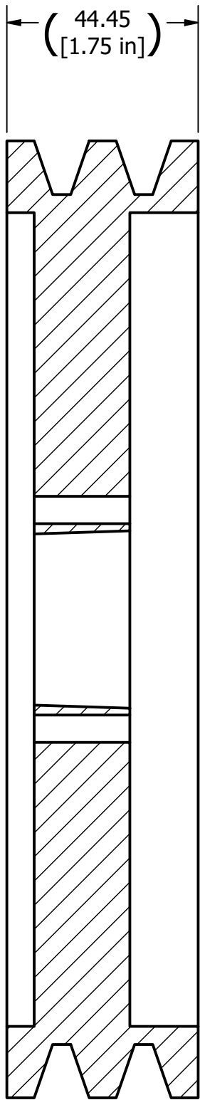
SECTION A-A
